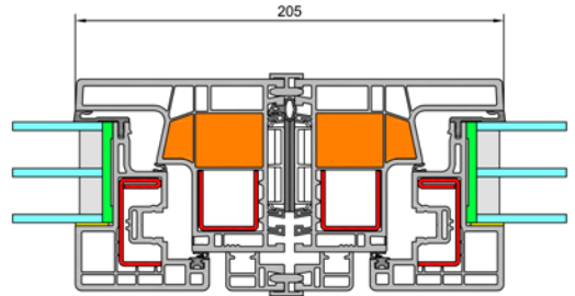
Schnitt Kopplung
