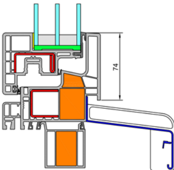
Schnitt Fußpunkt
