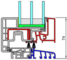
Schnitt Fenstertür
