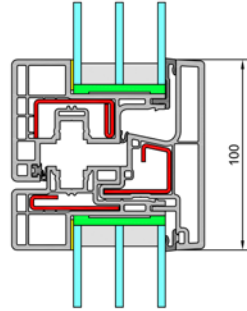
Schnitt Stulp/Pfosten
