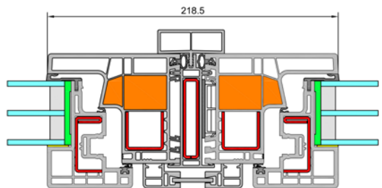
Schnitt Statikkopplung
