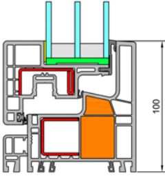
Grundschnitt GEALAN-KUBUS®
